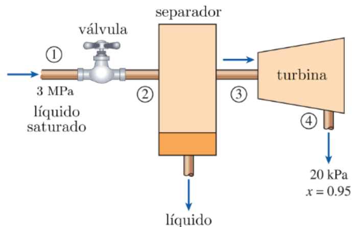
Figura 1. Planta geotérmica en estudio.
