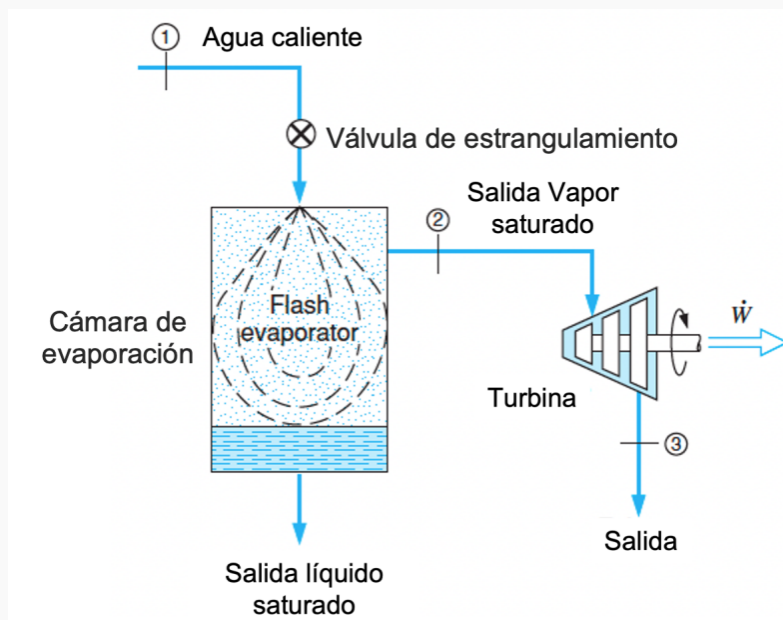
Figura 6. Sistema sobre fuente geotérmica en estudio.
